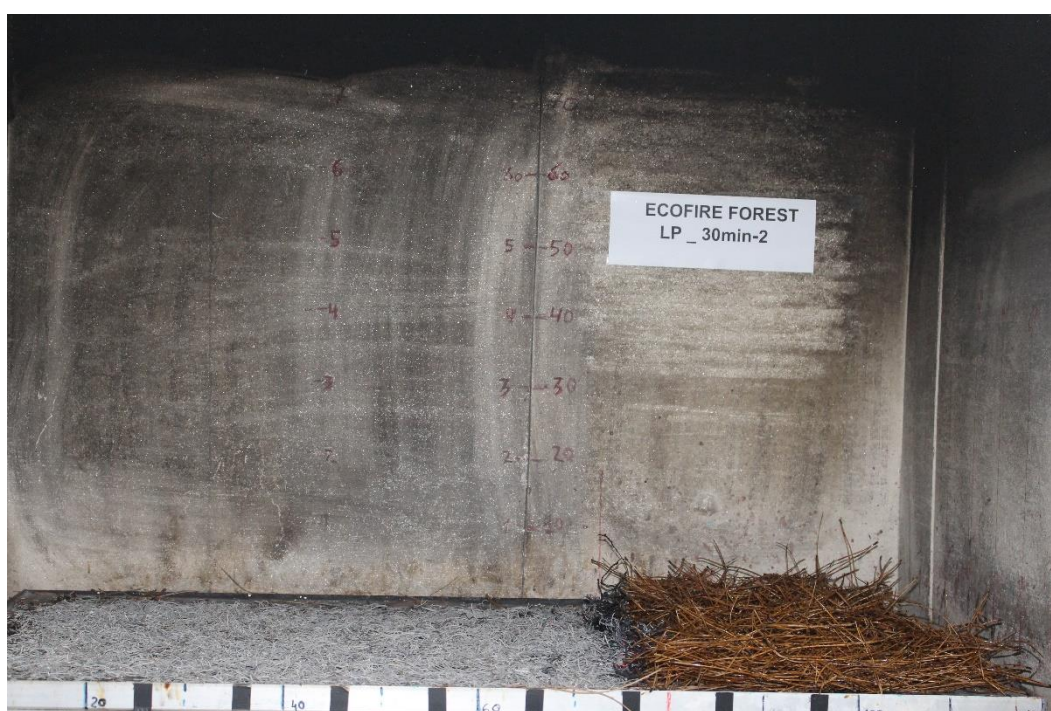
Fotografía nº 6.- Vista del residuo al final del ensayo, para el tratamiento 1 (30 minutos en estufa)
