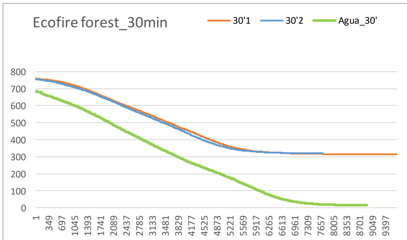
Gráfico n° 1: Curvas peso-tiempo de los ensayos realizados para el tratamiento 1 y el tratamiento con agua (30 minutos en estufa)
