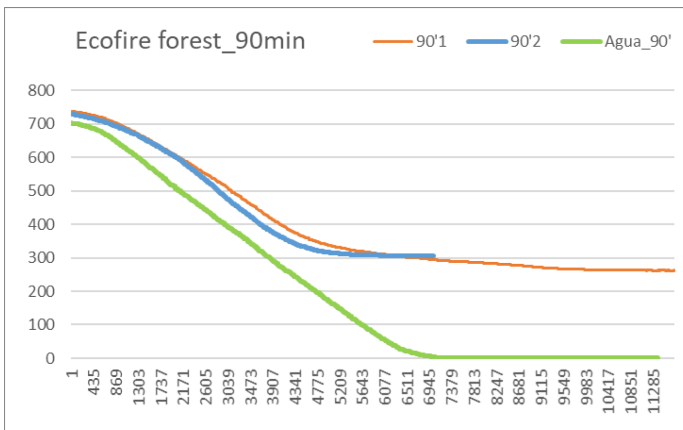
Gráfico n° 1: Curvas peso-tiempo de los ensayos realizados para el tratamiento 2 y el tratamiento con agua (90 minutos en estufa)
